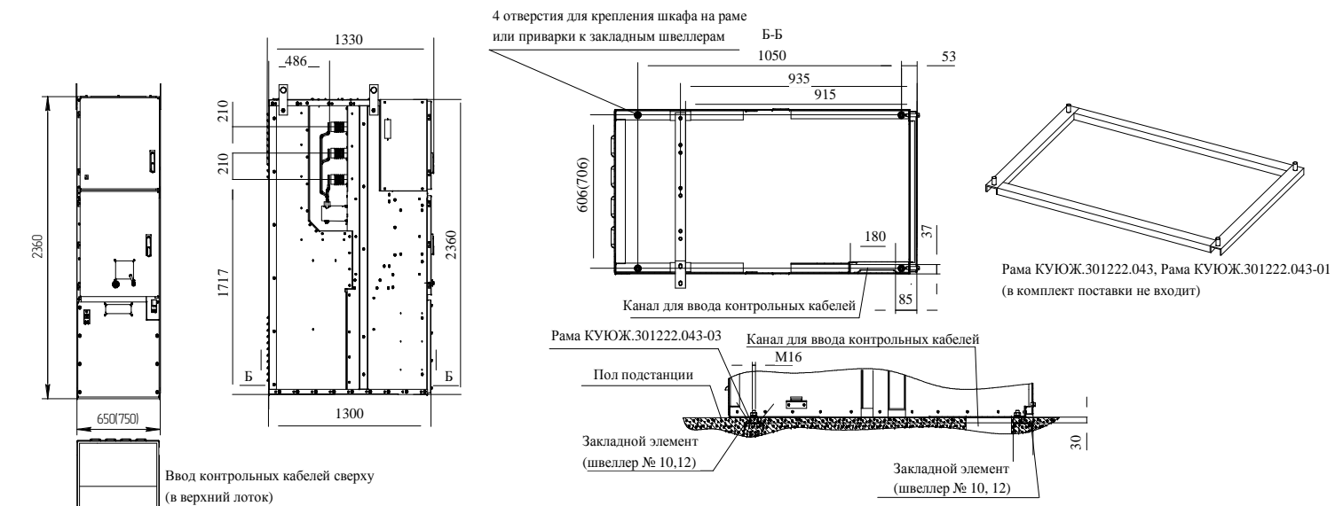
Рисунок Б.6 - Габаритные и установочные размеры шкафов КРУ для крепления их на фундаменте для схем от 300 до 320
