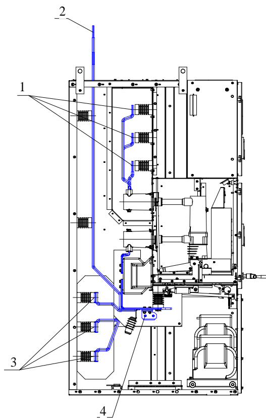
Рисунок X.3 - Точки измерения электрических сопротивлений главной цепи шкафа КРУ типа КС-10-(001-061) с шинным вводом
