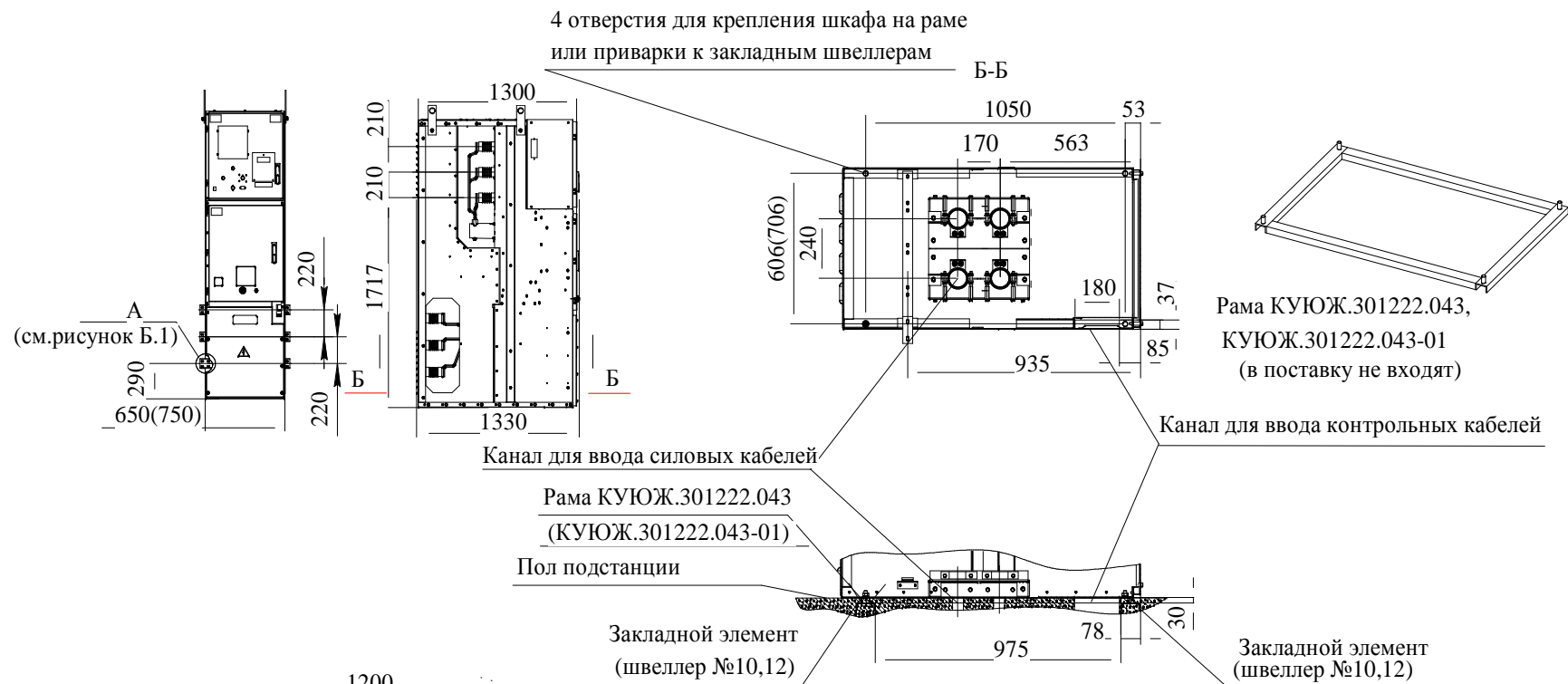
Рисунок Б.2 - Габаритные и установочные размеры шкафов КРУ типа КС-10-20(31,5)-1000 (1600) для крепления их на фундаменте для схем (013 - 020); (025 - 032); (037 - 042); (051 - 058); (100 - 101)
