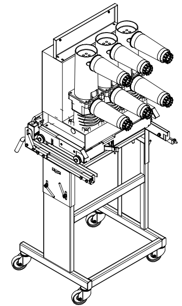
Рисунок М.3- Выкатной элемент на инвентарной тележке
