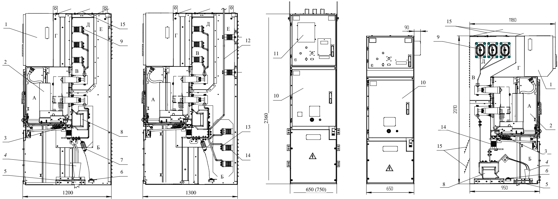
Шкаф КРУ КС-10-20(31,5)-1000(1600) с кабельным вводом.
