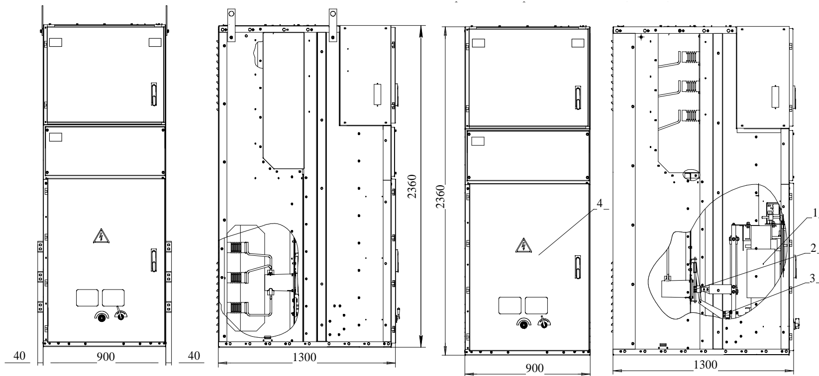
Рисунок Е.1 - Схематическое изображение шкафа КРУ типа КС-10-(201-203)
