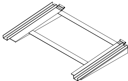
Рисунок Е.3 - Пандус КУЮЖ.301224.009 (входит в комплект поставки)
