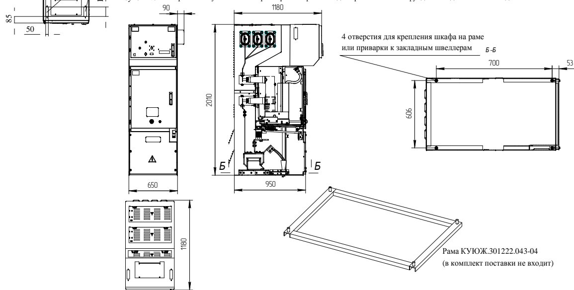
Рисунок Б.7 - Габаритные и установочные размеры шкафов КРУ типа КС-10-20-1000(1250)-60(61) для крепления их на фундаменте для схем 033; 034; 035; 036 Остальное см. рисунок Б.6
