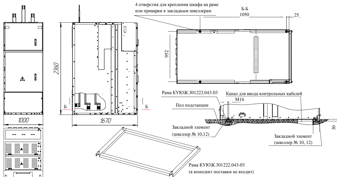
Рисунок Б.8- Габаритные и установочные размеры шкафов КРУ типа КС-10-40-3150 для крепления их на фундаменте для схем 006; 008; 050
