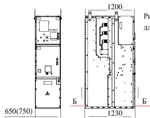
Рисунок Б.3 - Габаритные и установочные размеры шкафов КРУ типа КС-10-20(31,5)-1000 (1600) для крепления их на фундаменте для схем (021 - 024); (033 - 036) Остальное см. рисунок Б.2
