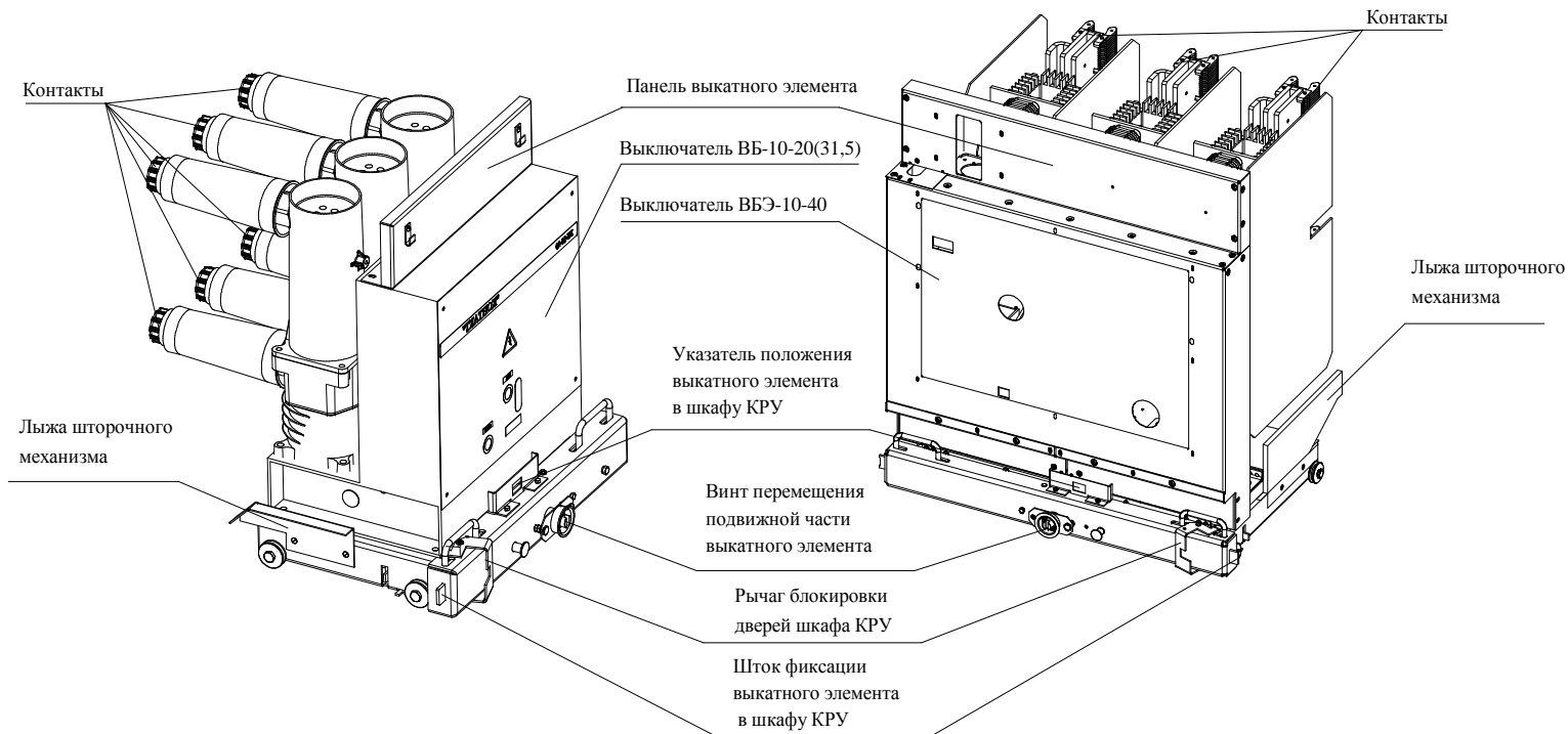
Рисунок М.2 - Схематическое изображение выкатного элемента шкафа КРУ типа КС-10-40-3150
