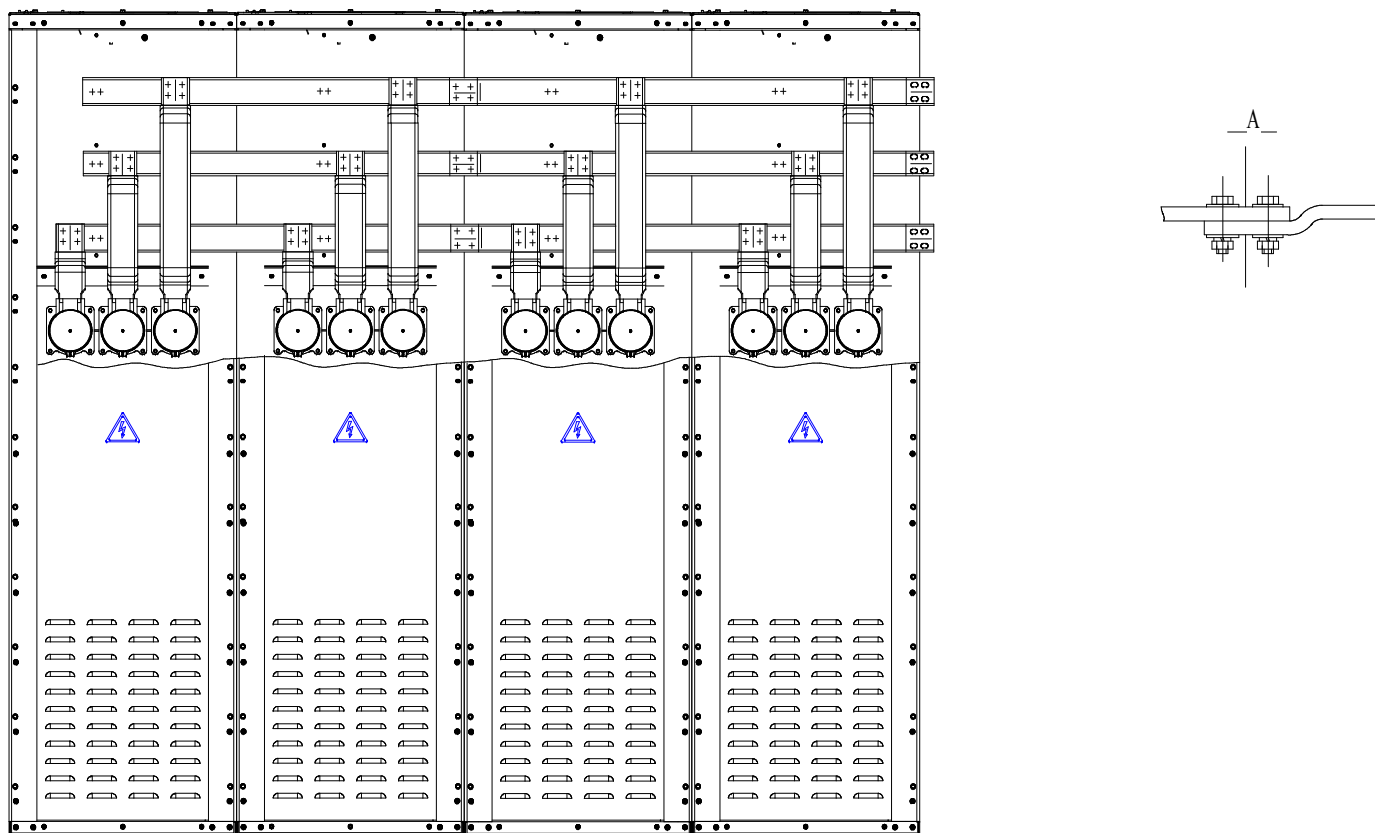
Схема монтажа сборных шин шкафов КРУ (вид сверху)
