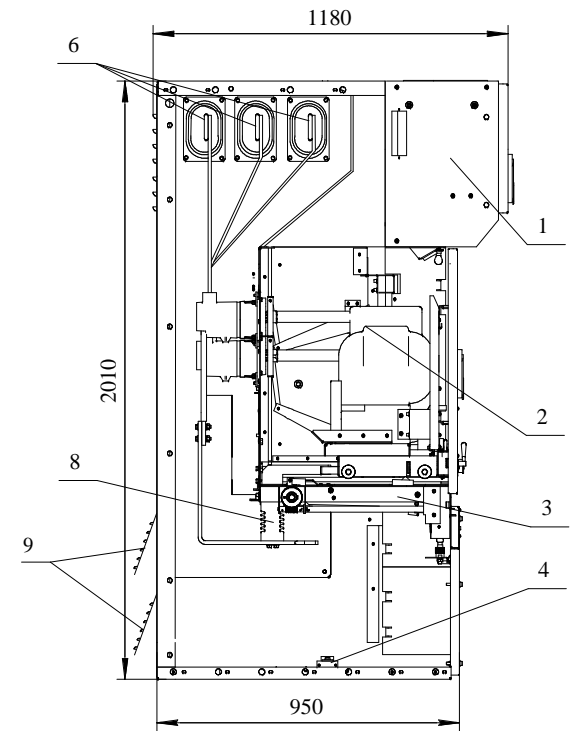
Шкаф КРУ КС-10М-(300-303)-20-1000 с трансформаторами напряжения.
