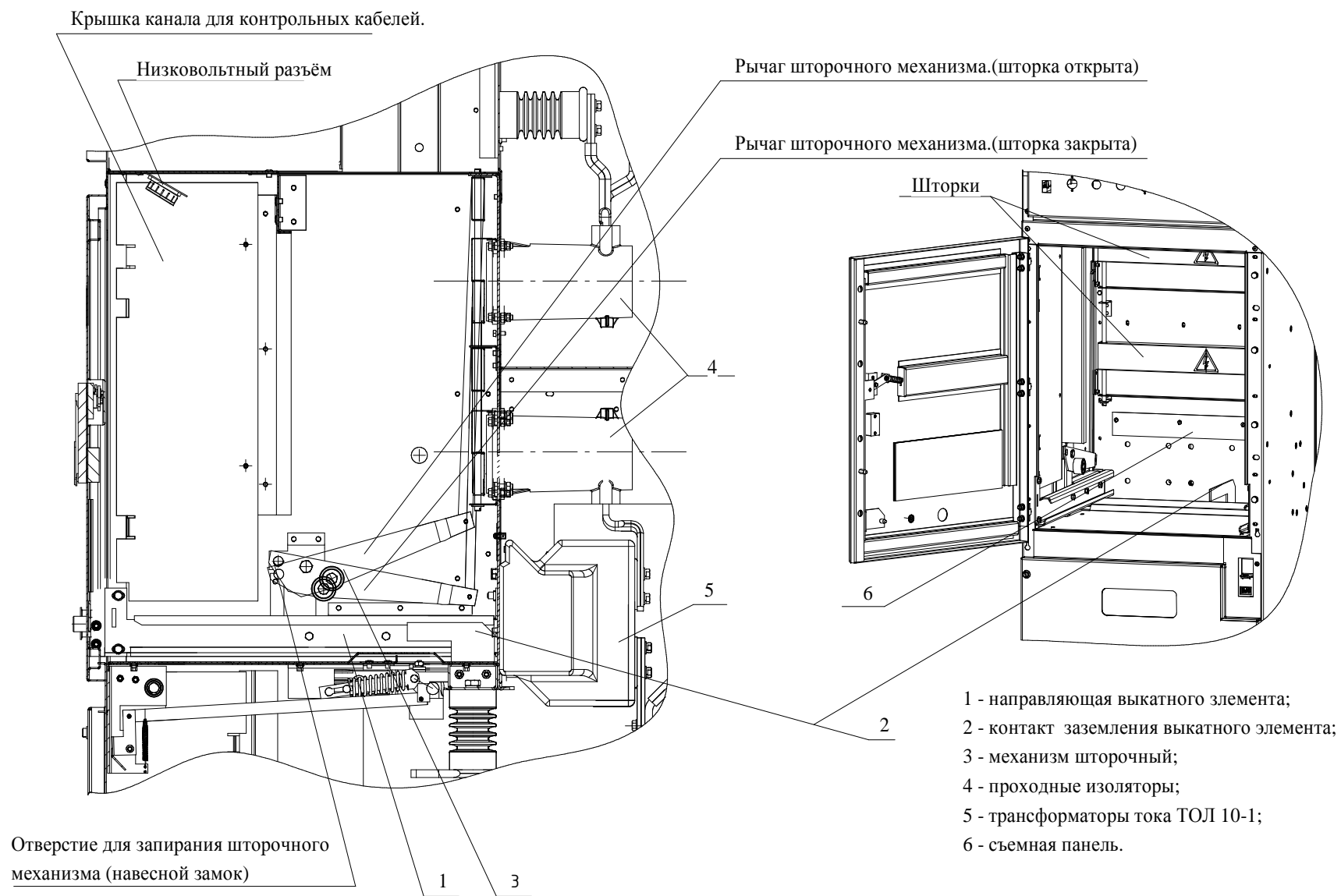
Рисунок Л.1 Схематическое изображение отсека выкатного элемента шкафов КРУ типа КС-10-20(31,5)-1000(1600)
