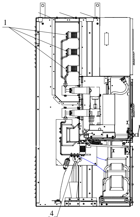
Рисунок X.4 - Точки измерения электрических сопротивлений главной цепи шкафа КРУ типа КС-10-(001-061) с кабельным вводом
