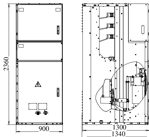
Рисунок Б.5 - Габаритные и установочные размеры шкафов КРУ для крепления их на фундаменте для схемы 200 (без линейных шин)
