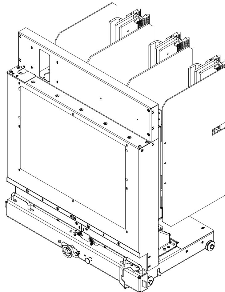
Рисунок Н.2 Схематическое изображение выкатного элемента шкафа КРУ типа КС-10-40-3150-(100-101)
