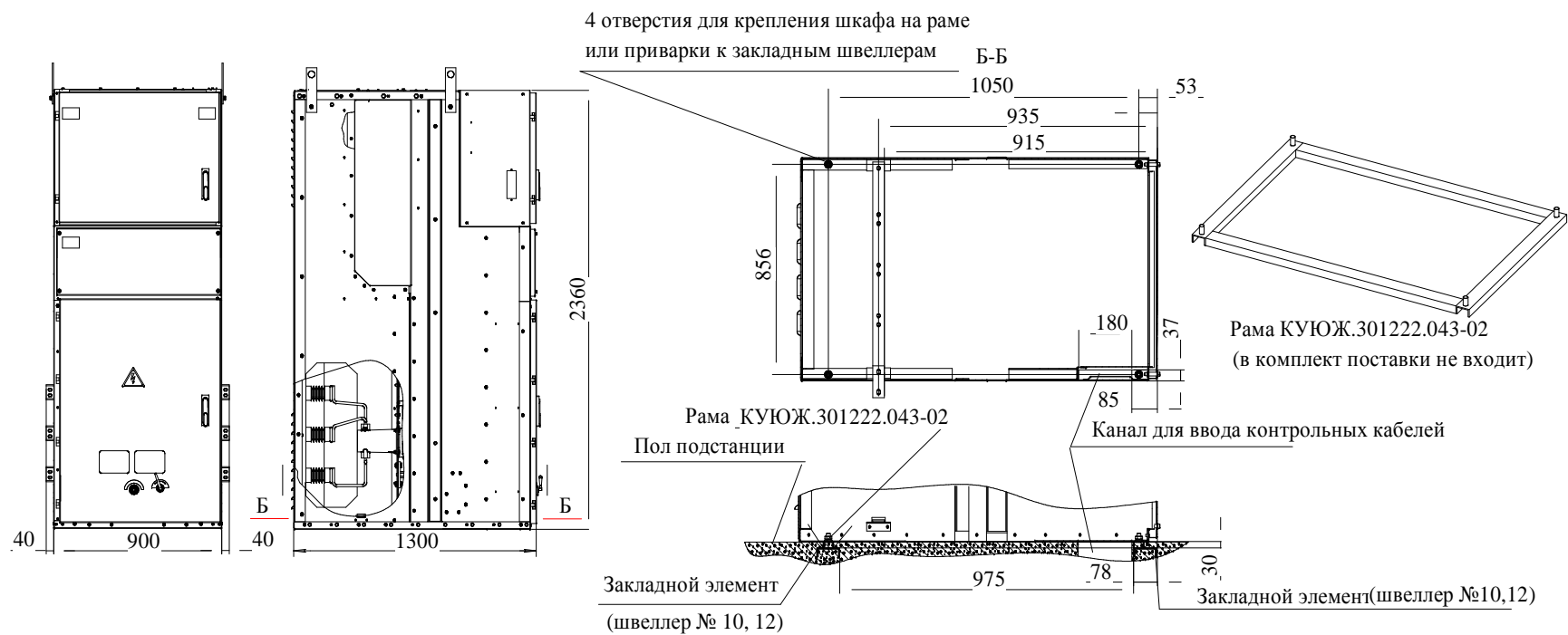
Рисунок Б.4 - Габаритные и установочные размеры шкафов КРУ для крепления их на фундаменте для схем от 201 до 203
