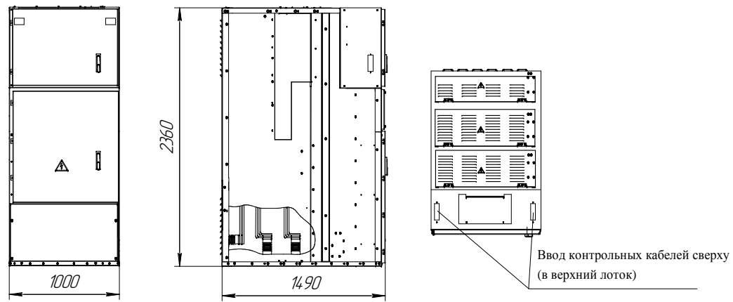
Рисунок Б.9- Габаритные и установочные размеры шкафов КРУ типа КС-10-40-3150 для крепления их на фундаменте для схем 027; 031; 057; 100; 101 Остальное см. рисунок Б.8
