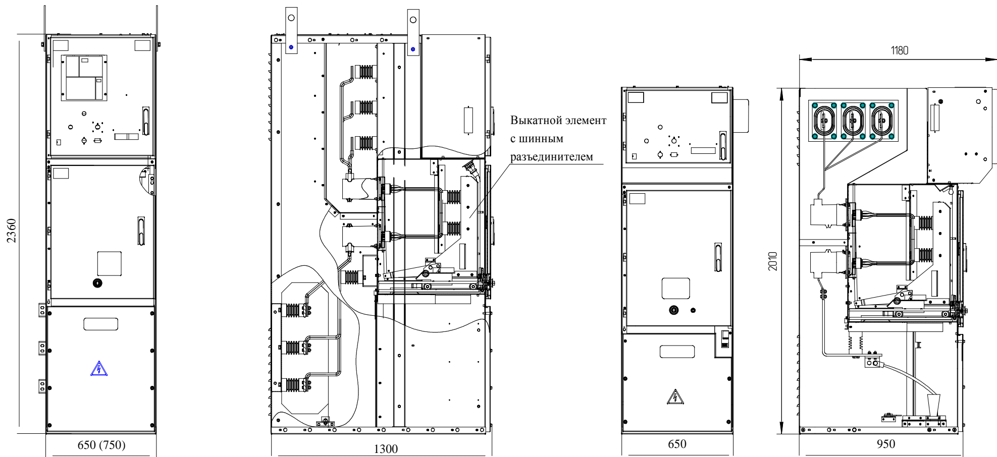
Схематическое изображение шкафа КРУ типа КС-10-20(31,5)-1600-(100-101)
